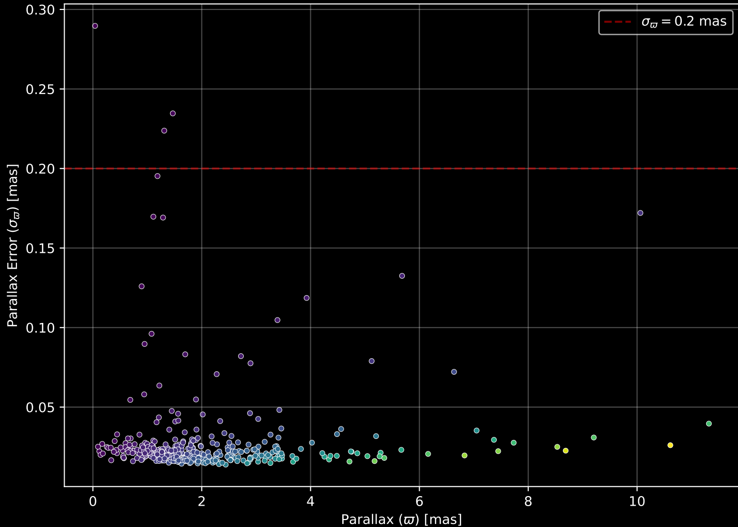
GALAH DR4 Field: [6693] Parallax Quality (n= 387)
