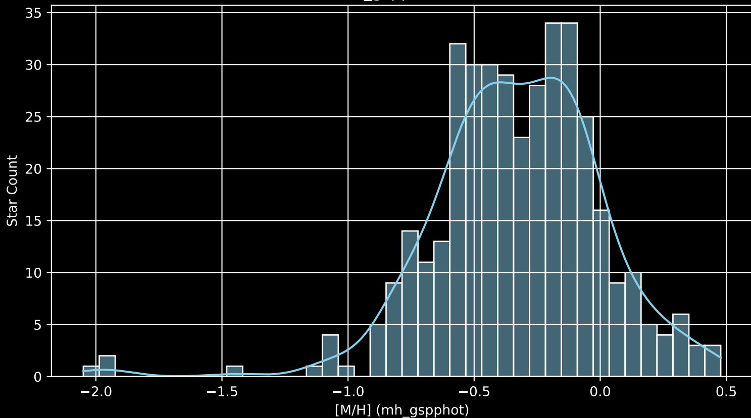
GALAH DR4 Field: [6693] [M/H] (mh_gspphot) (n= 383)
