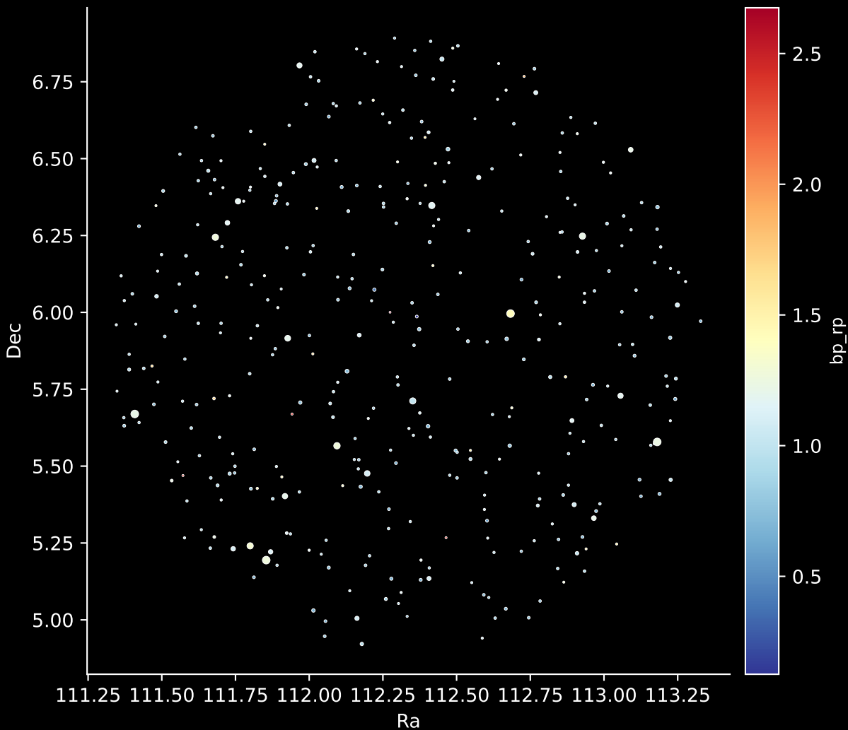
GALAH DR4 Field: [6693] Stars: 387
