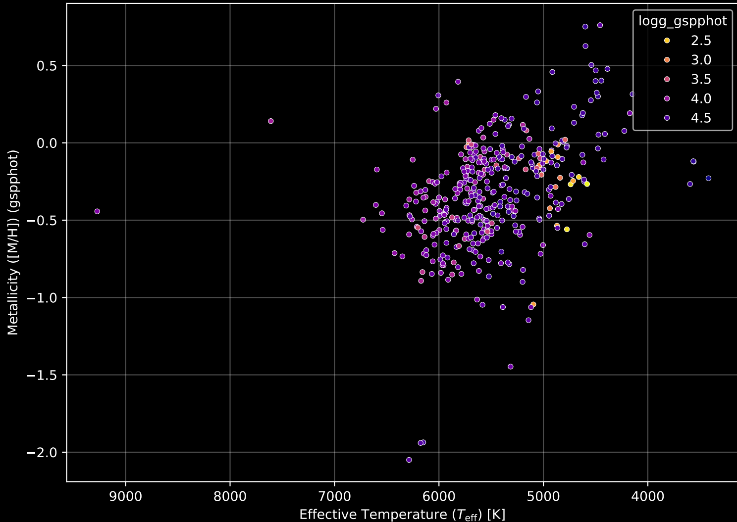
GALAH DR4 Field: [6693] Stellar Population Parameters (n= 387)
