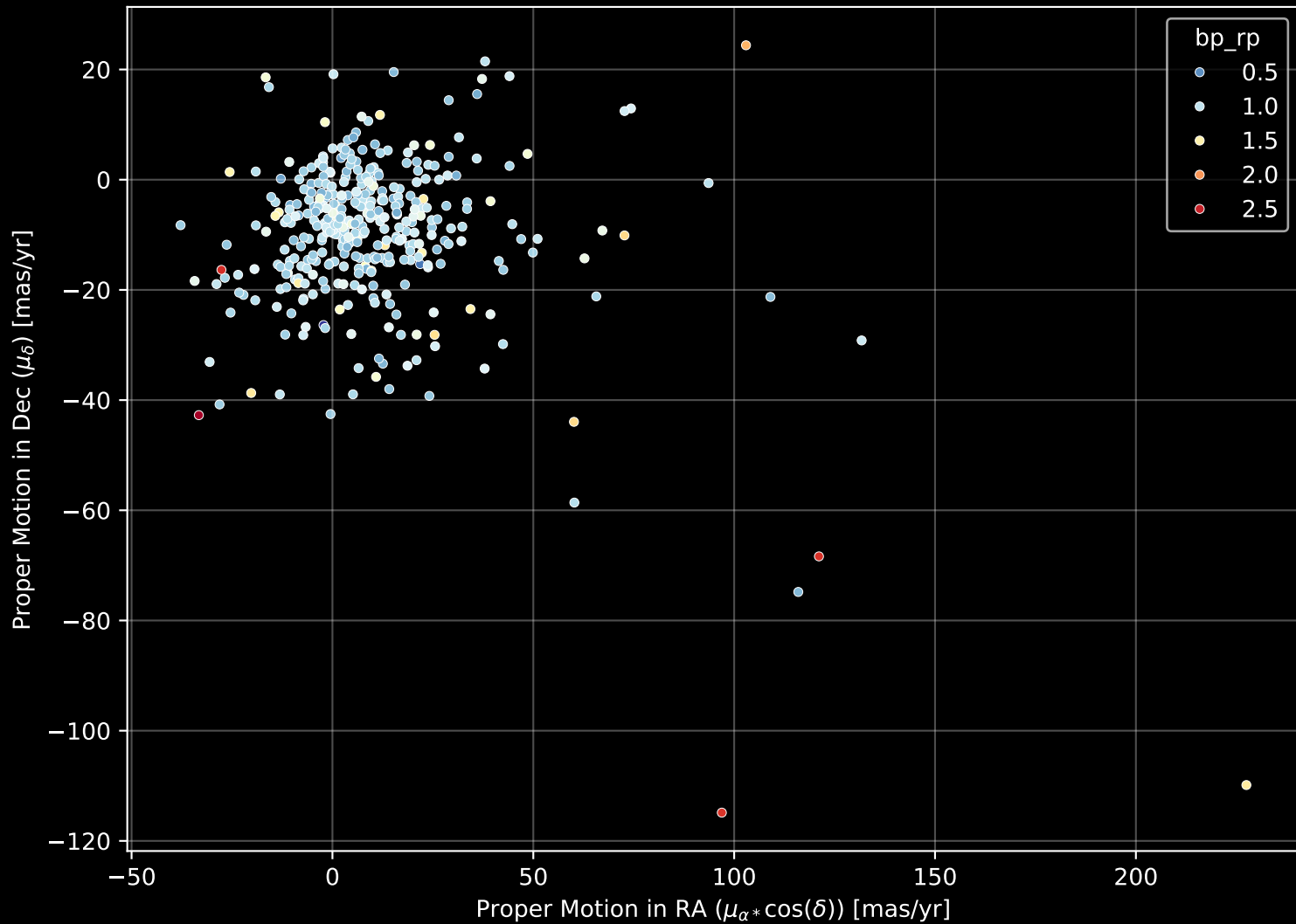
GALAH DR4 Field: [6693] Proper Motion Diagram (n= 387)
